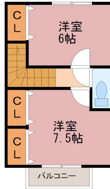
2F
